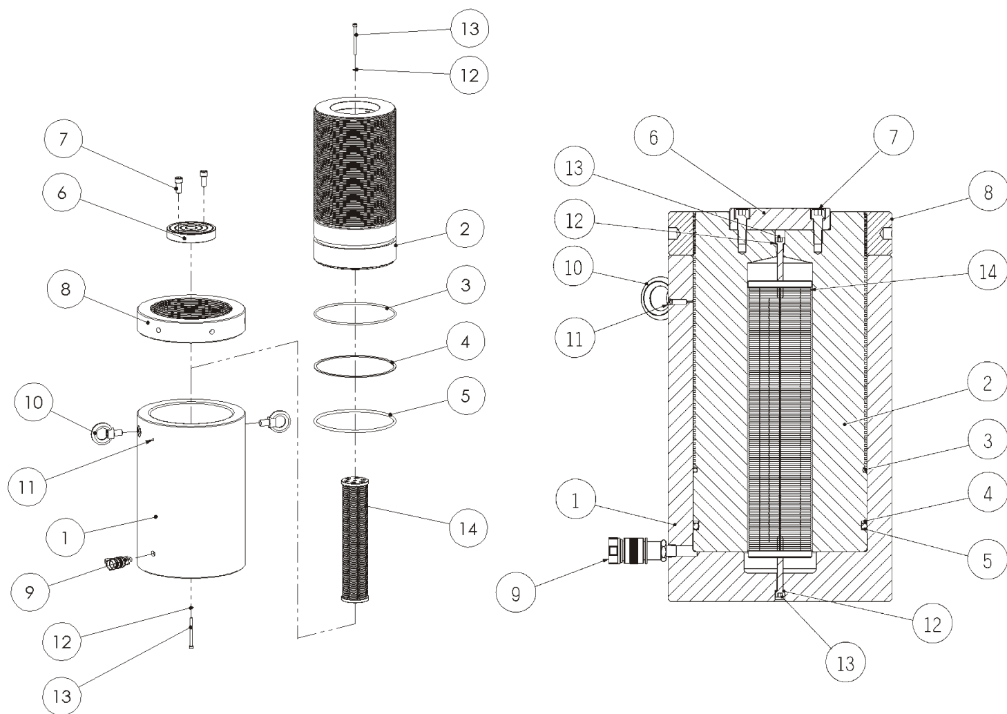
Q1-單動高噸位鎖帽CSLL型-彈簧 (CSLL-30012XF)
