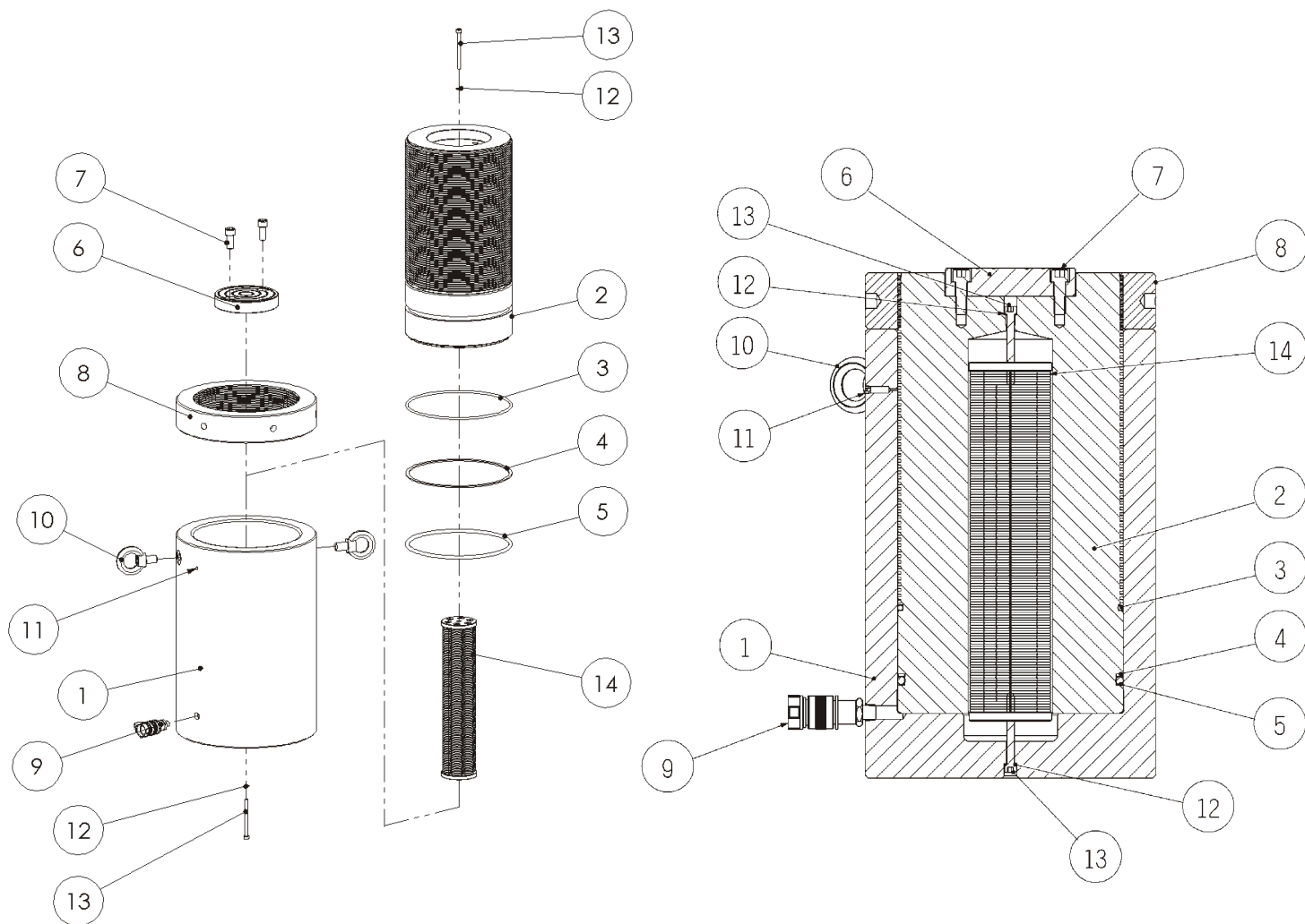
Q1-單動高噸位鎖帽CSLL型-彈簧 (CSLL-40012XF)
