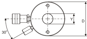
缸底墊塊前底座螺孔圖示
