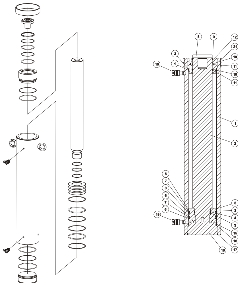
M-雙動/塞底/主軸內牙/上螺帽/溝槽墊塊型(RSR-40018)
