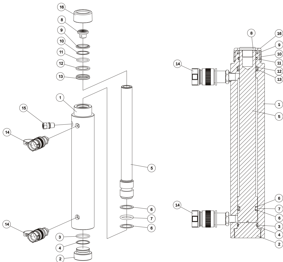
L-雙動/塞底/主軸內牙/溝槽墊塊型(RSR-1012)
