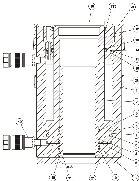
H1-雙動/中空RSRH型(RSRH-603)
