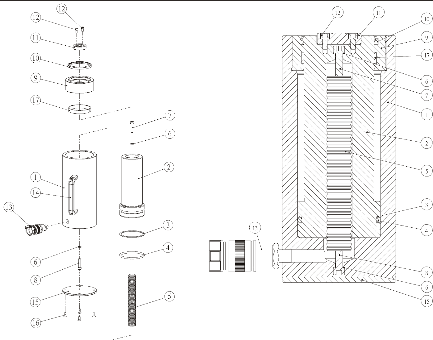
F-鋁合金RSAC型(RSAC-306)
