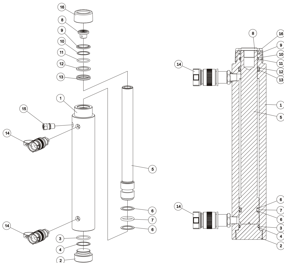
L-雙動/塞底/主軸內牙/溝槽墊塊型(RSR-1010)
