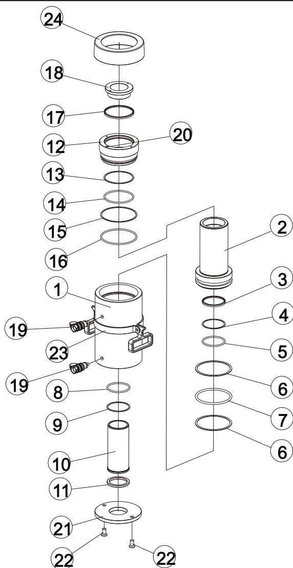
H1-雙動/中空RSRH型(RSRH-6010)
